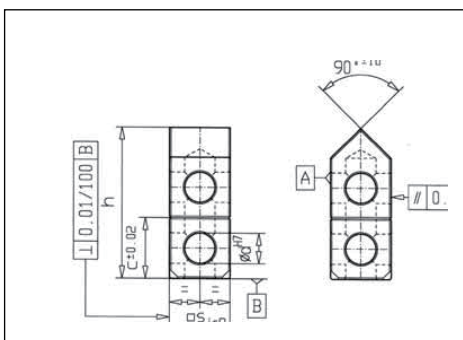
倒V支撑件 90° Form 2
