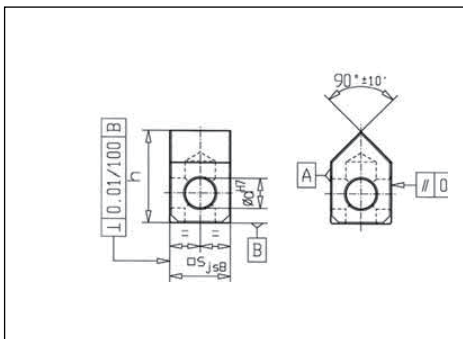
倒V支撑件 90° Form 1
