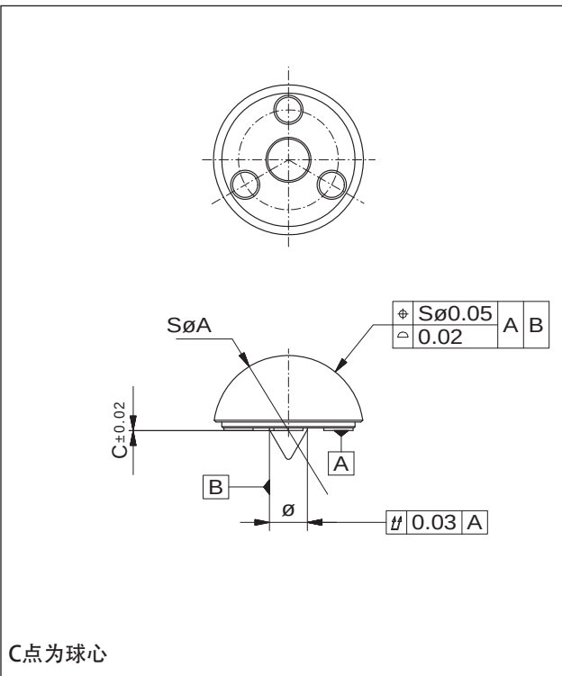
Fixinspect "R" 测量附件的形位公差
