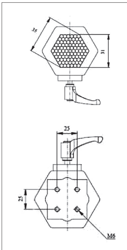
俯视图
