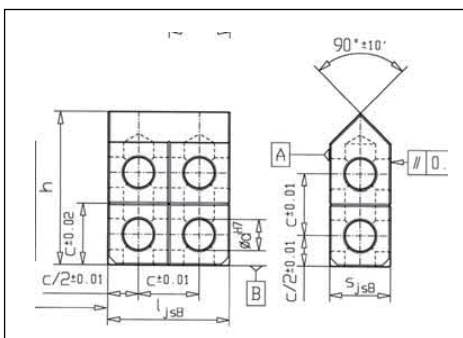
倒V支撑件 90° Form 3
