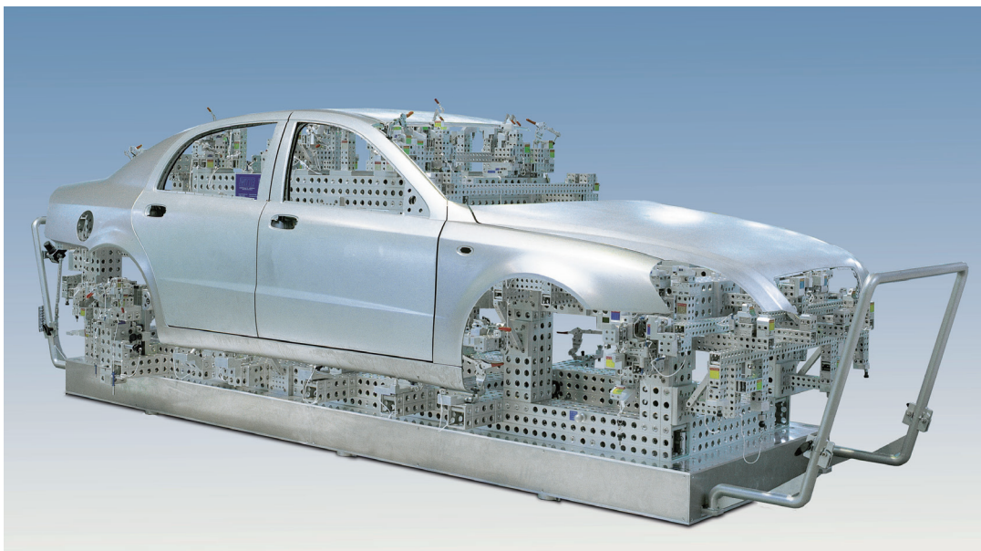
外精测样架用于匹配车身外覆盖件,模拟总装状态
