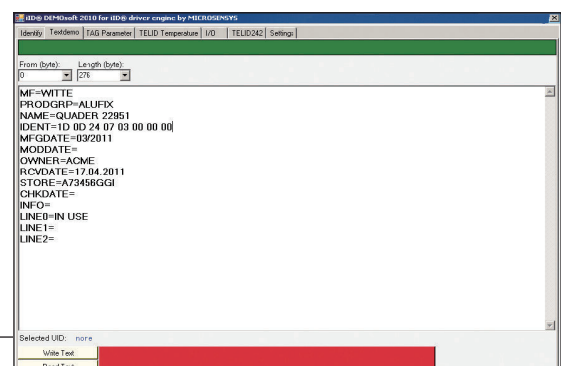
RFID芯片中独立存放的信息
