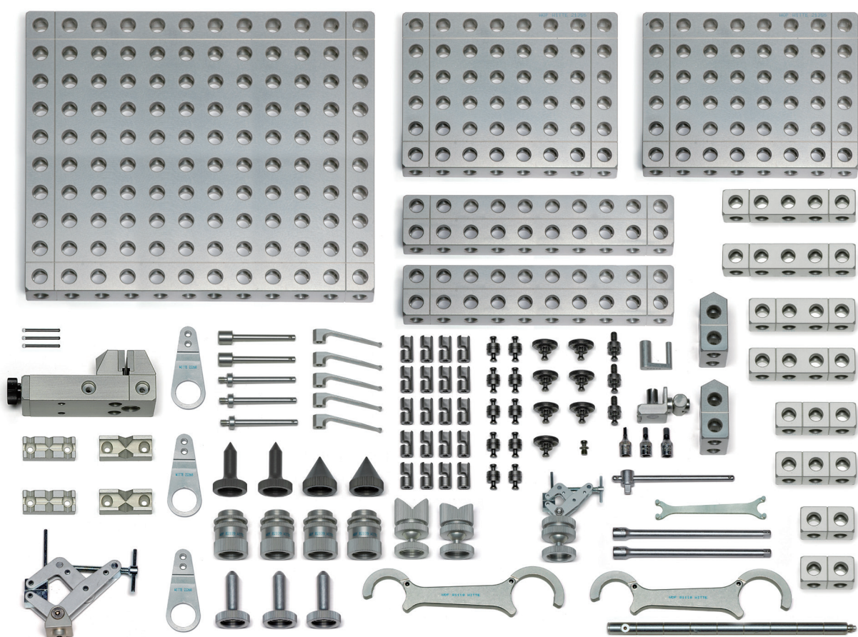
#106526 套件 3 Alufix 25 (106-pcs), 12,6kg
