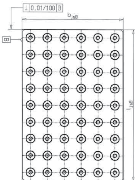
2小工件支架固定在单面孔基板上
